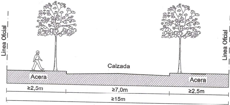
PERFIL TIPICO VIA DE SERVICIO
